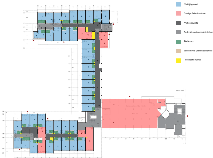
Plattegrond BG
